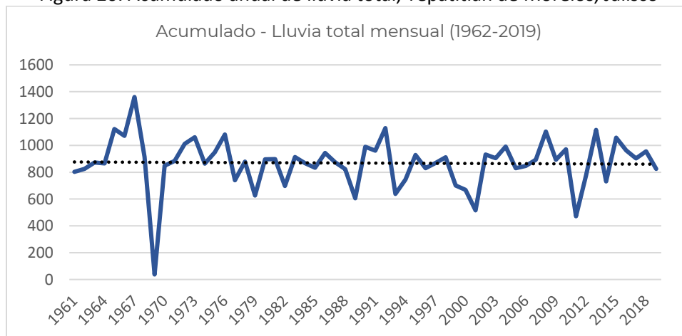
Figura 20. Acumulado anual de lluvia total, Tepatitlán de Morelos, Jalisco
