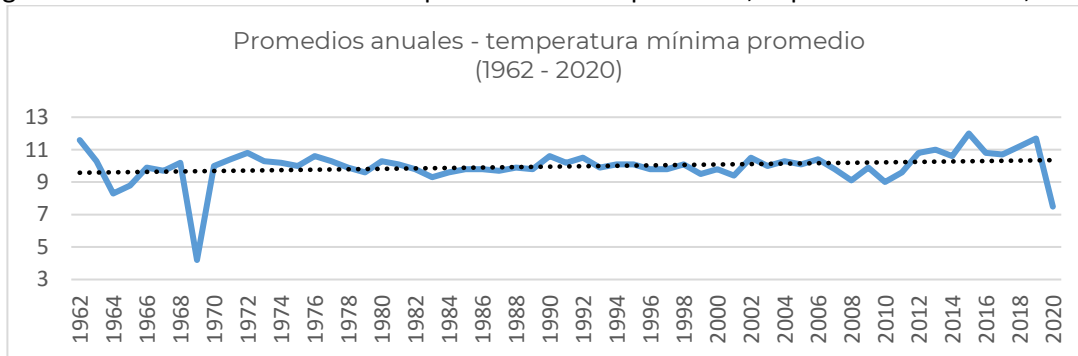
Figura 18. Promedios anuales de temperatura mínima promedio, Tepatitlán de Morelos, Jalisco
