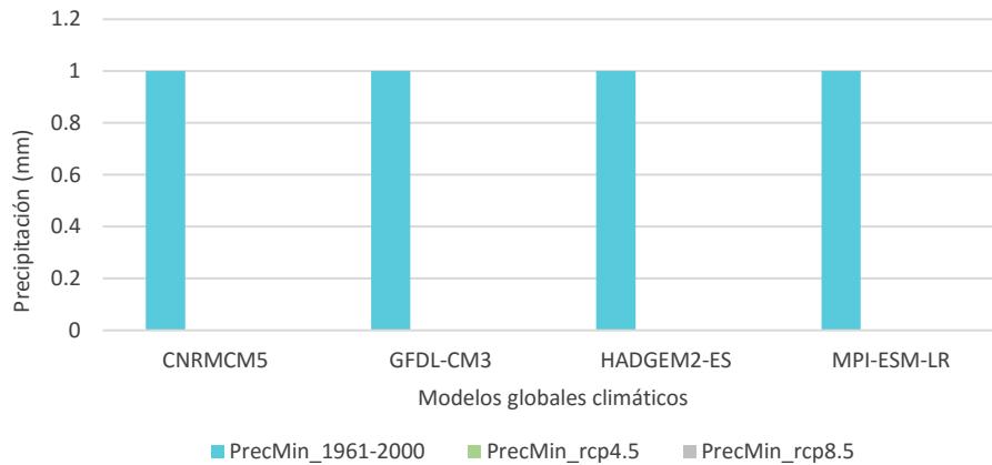
Figura 26. Proyecciones climáticas; Comparativo de precipitación mínima del periodo 1961-2000 con proyección 2015-2039 del mes de marzo con los cuatro MGC y con RCP 4.5 y 8.5.
