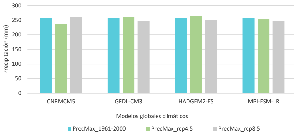
Figura 27. Proyecciones climáticas; Comparativo de precipitación máxima del periodo 1961-2000 con proyección 2015-2039 del mes de julio con los cuatro MGC y con RCP 4.5 y 8.5.
