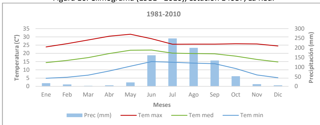
Figura 16. Climograma (1981 - 2010), estación 14087, La Red.
