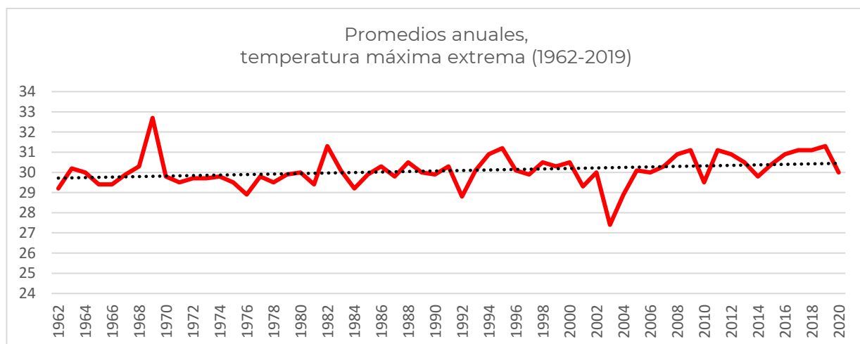
Figura 29. Promedios anuales de temperatura máxima extrema, Tepatitlán de Morelos, Jalisco
