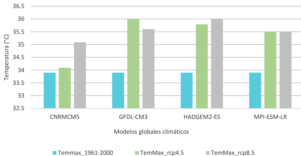
Figura 25. Proyecciones climáticas; Comparativo de temperatura máxima del periodo 1961-2000 con proyección 2015-2039 del mes de mayo con los cuatro MGC y con RCP 4.5 y 8.5.
