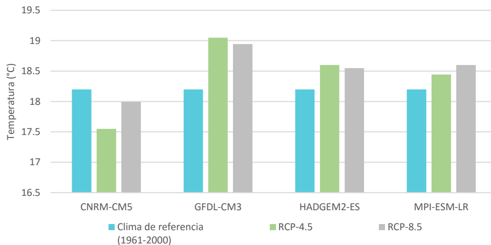
Figura 24. Proyecciones climáticas; Comparativo de temperatura media del periodo 1961-2000 con proyección 2015-2039 del mes de julio con los cuatro MGC y con RCP 4.5 y 8.5.
