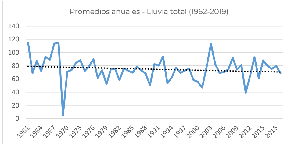
Figura 21. Promedios anuales de lluvia total, Tepatitlán de Morelos, Jalisco
