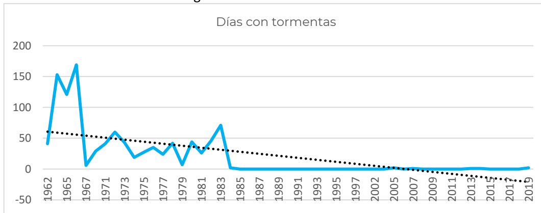
Figura 28. Días con tormentas.
